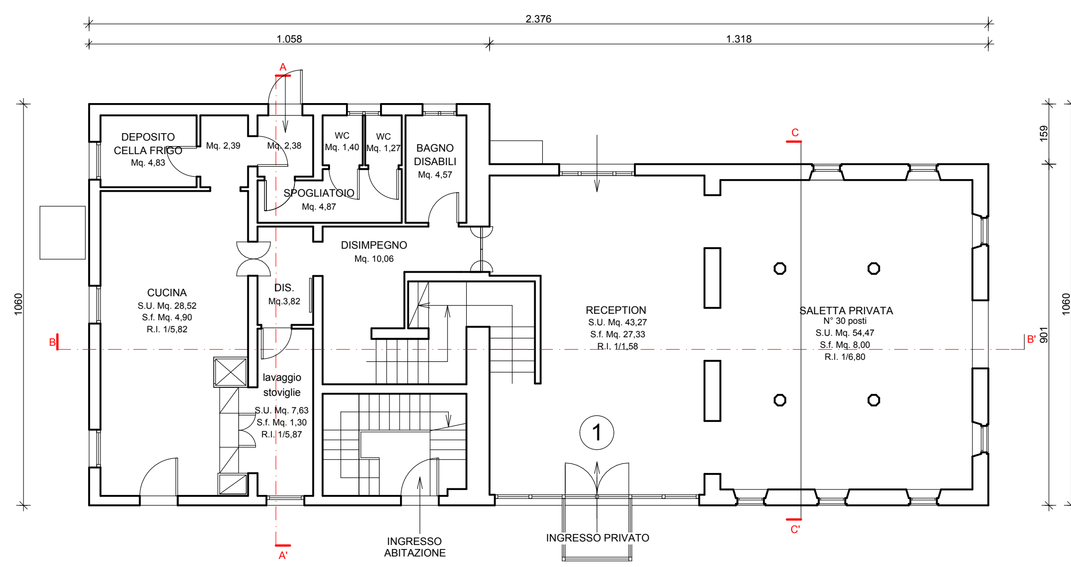
PIANTA PIANO TERRA - FABBRICATO 1
