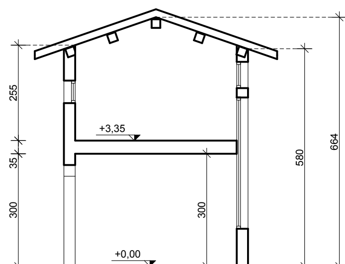
SEZIONE B - B' - FABBRICATO 2
