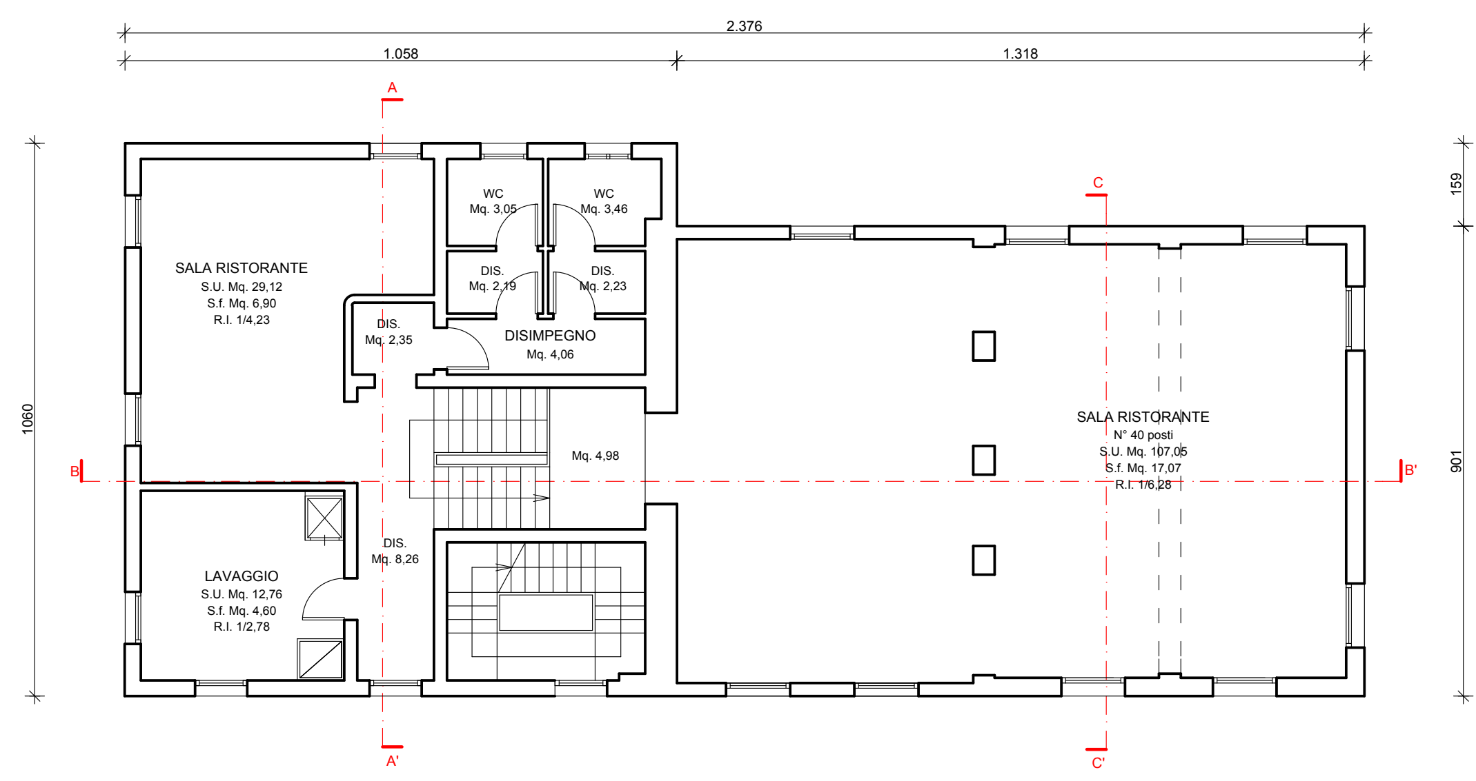
PIANTA PIANO PRIMO - FABBRICATO 1
