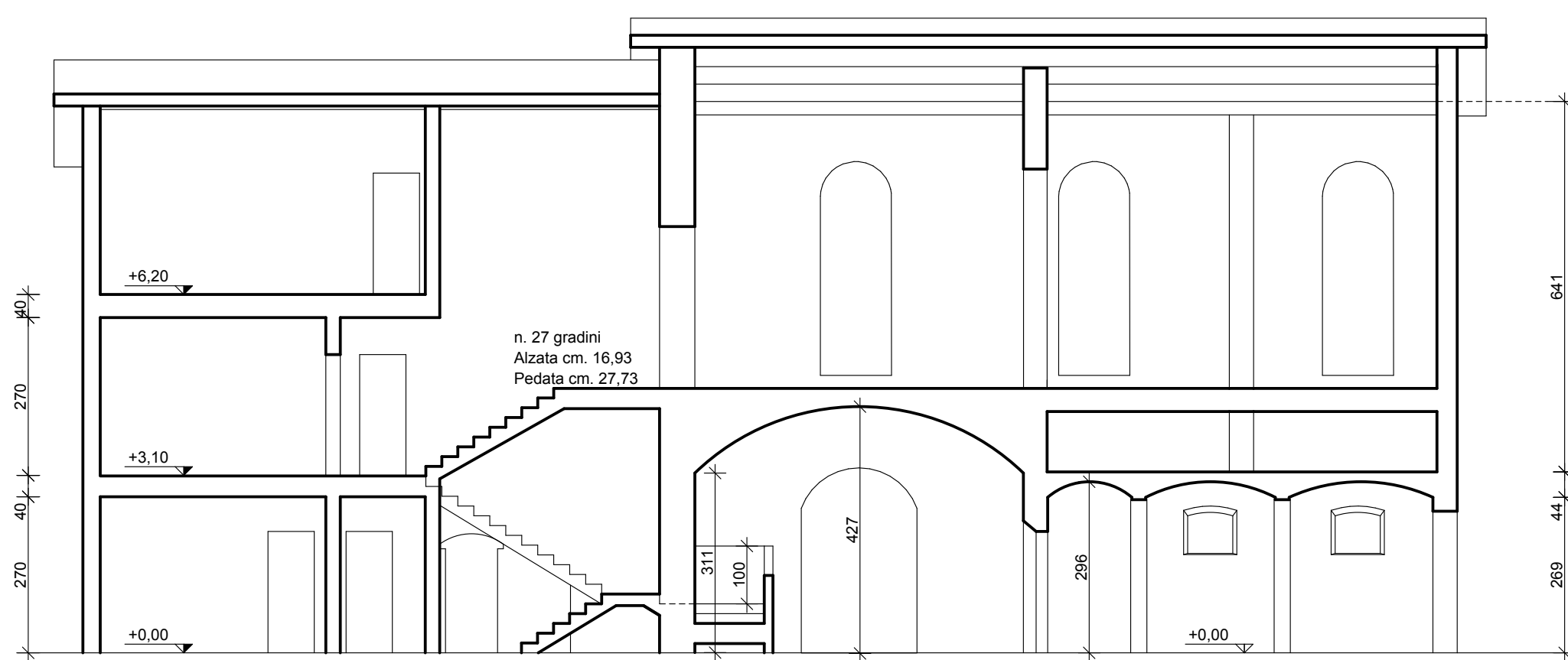
SEZIONE B - B' - FABBRICATO 1
