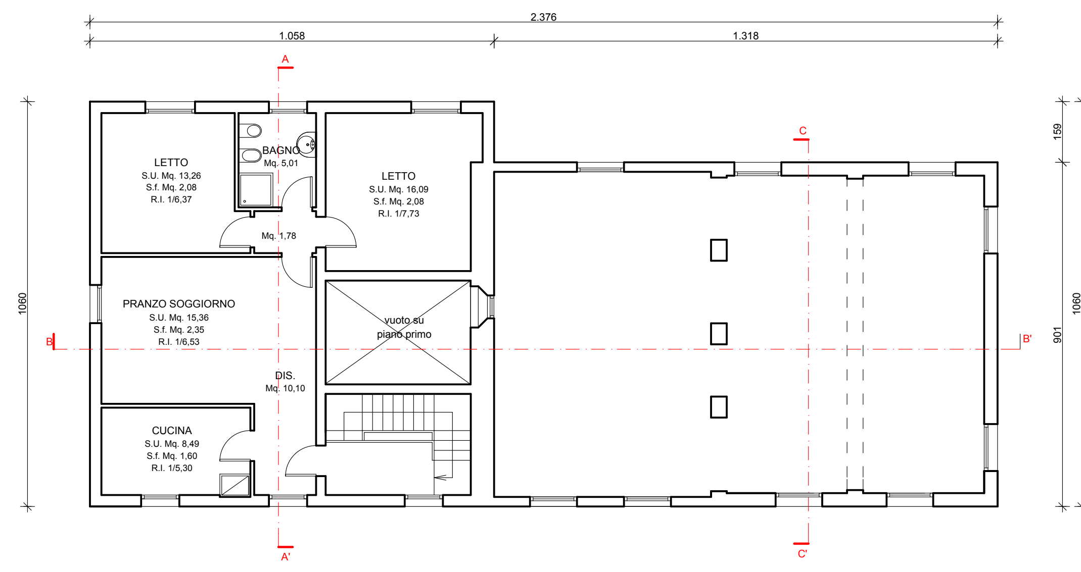
PIANTA PIANO SECONDO - FABBRICATO 1
