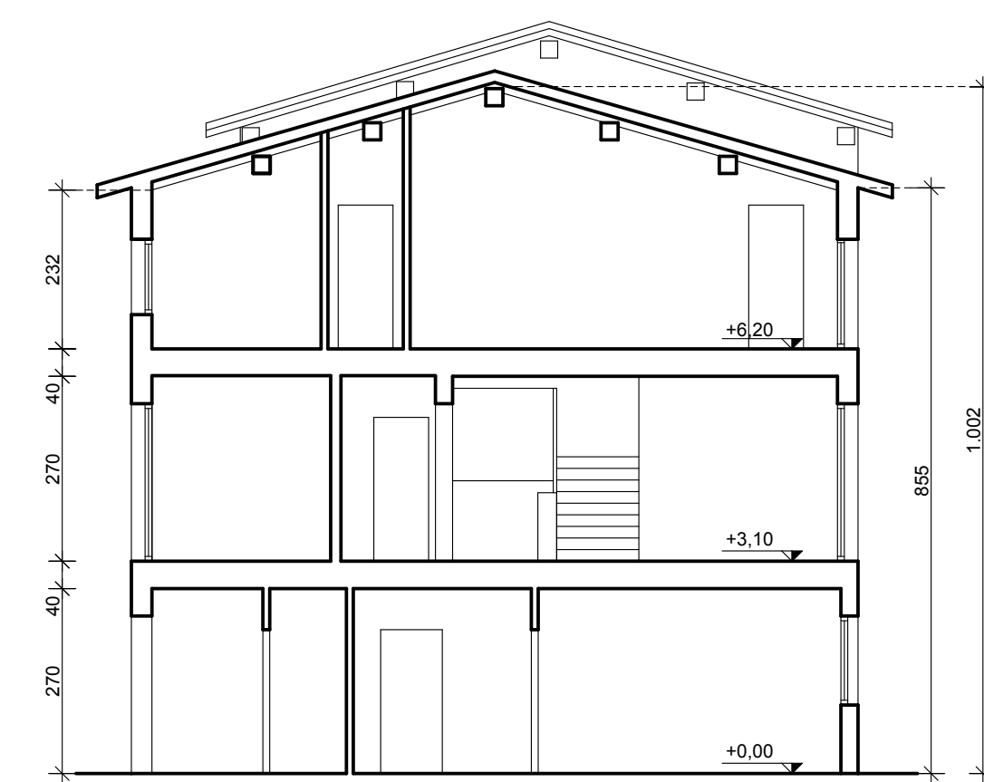
SEZIONE A - A' - FABBRICATO 1
