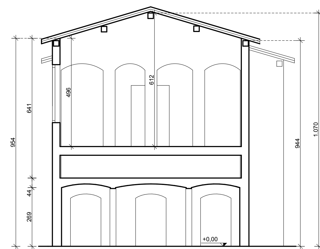
SEZIONE C - C' - FABBRICATO 1
