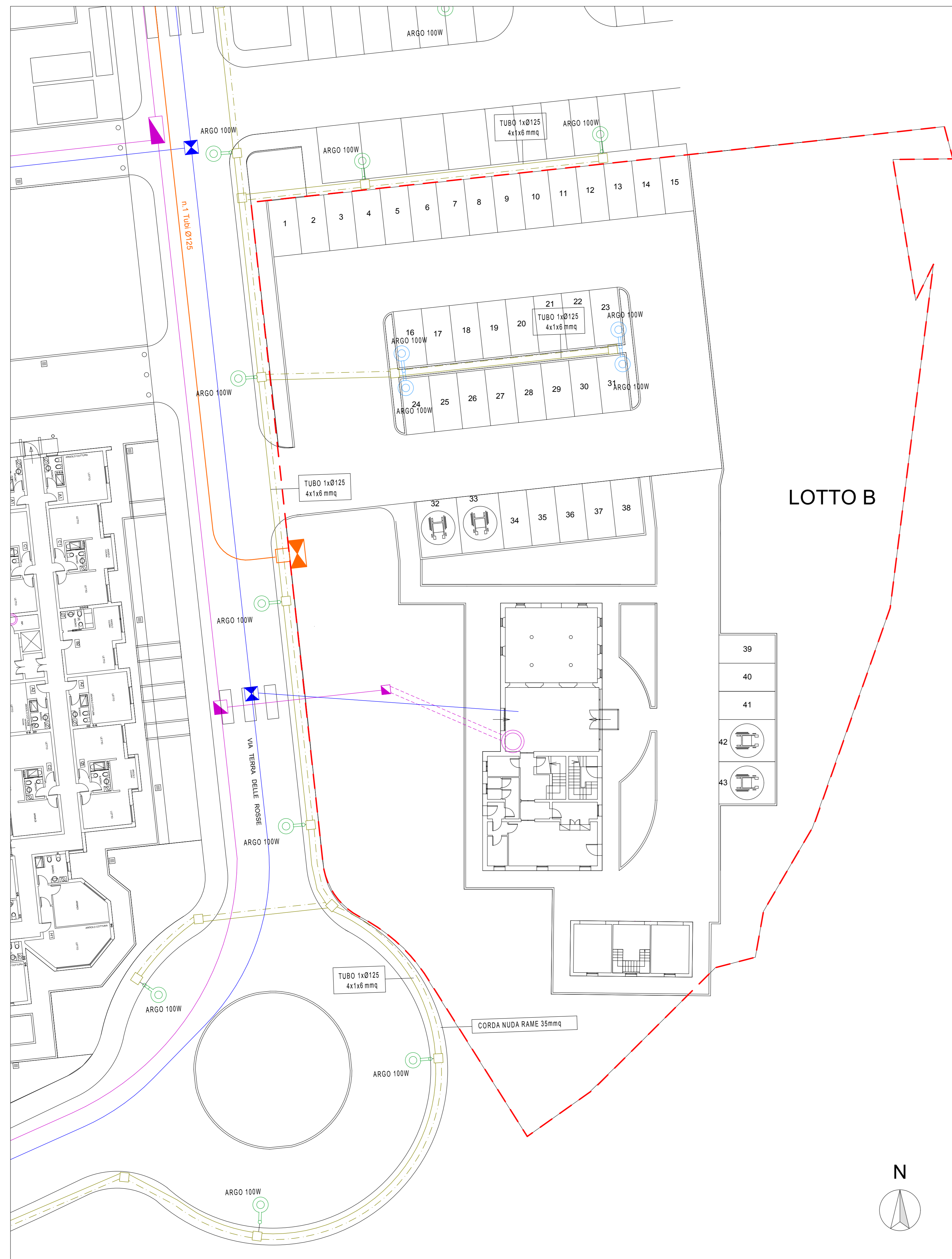
PLANIMETRIA ILLUMINAZIONE PUBBLICA, ENEL, TELECOM, FIBRE OTTICHE Scala 1:200
