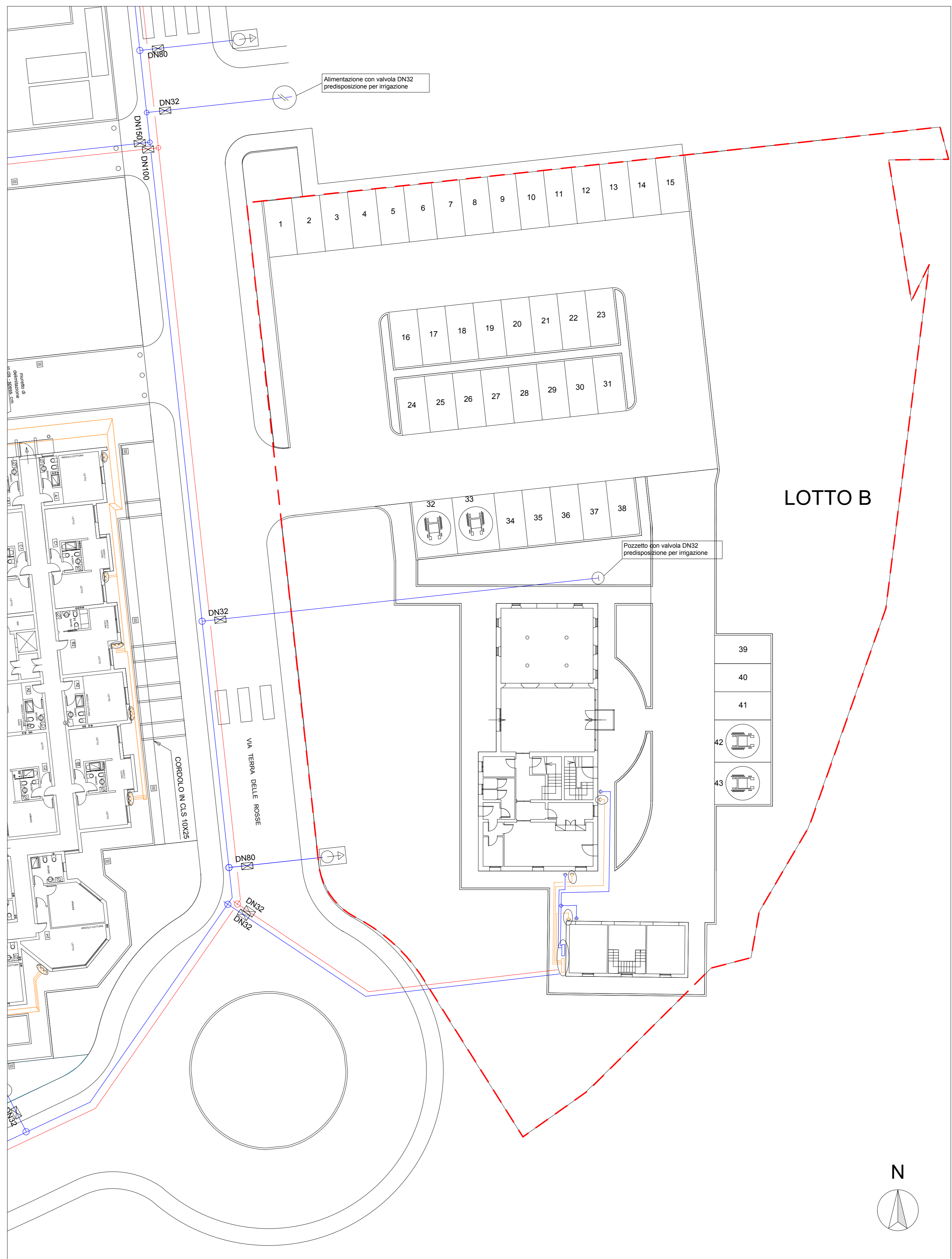
PLANIMETRIA IMPIANTI GAS E ACQUA Scala 1:200
