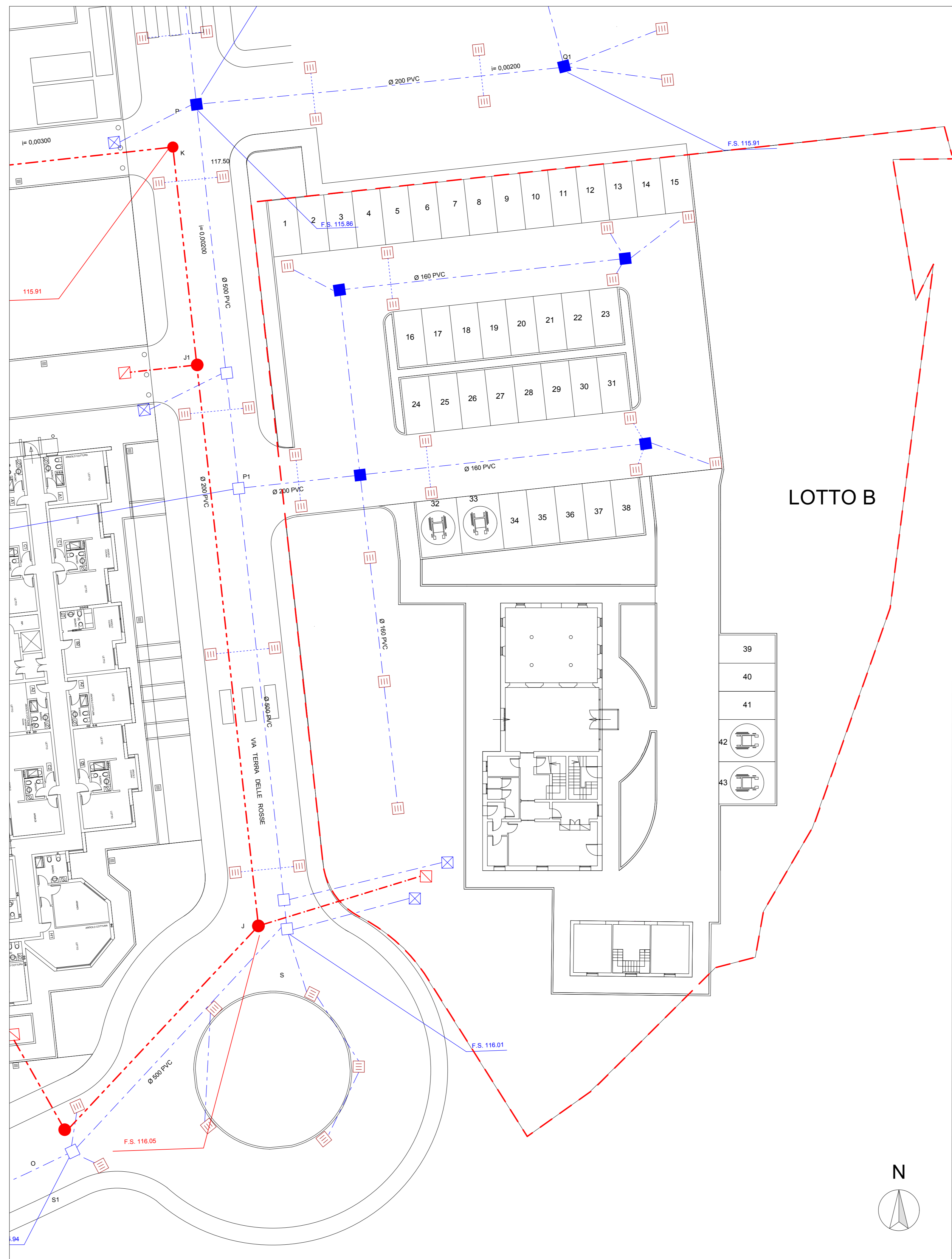
PLANIMETRIA RETE FOGNARIA Scala 1:200
