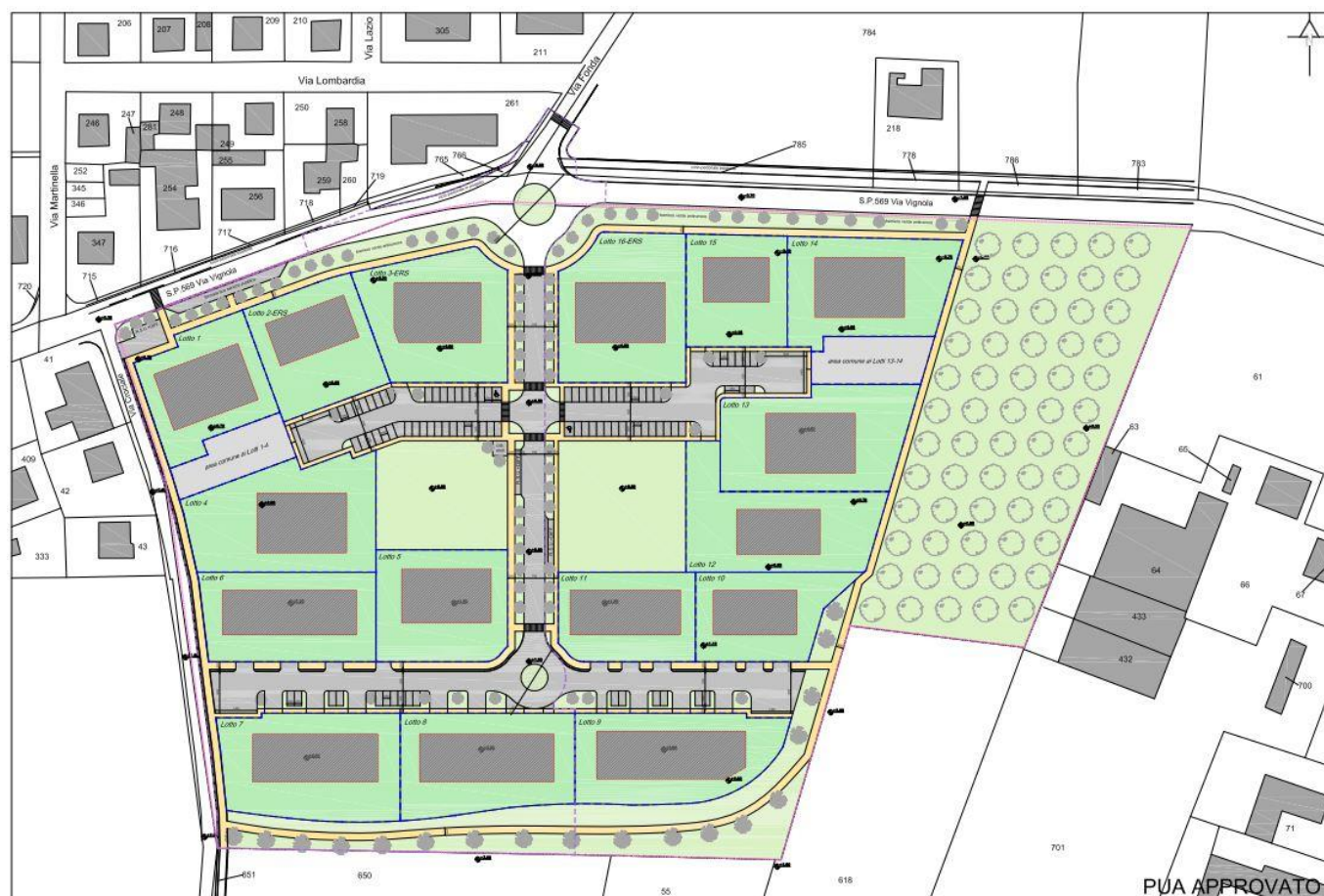
Fig. 1 – Planimetria PUA approvato (scala grafica).
